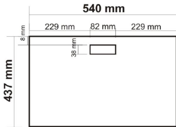
Upper Lid
