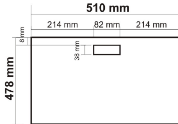
Bottom Lid
